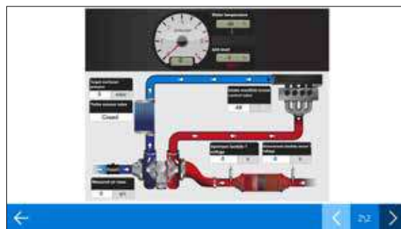
SISTEMA DE DOSIFICACIÓN DE AGENTES REDUCTORES
